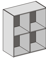
dělená skříňka 3 116 OD 800*400/780
